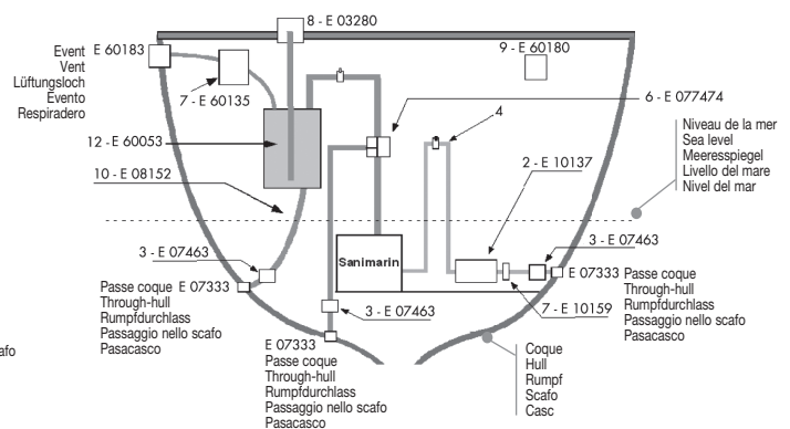
SCHEMA DE PRINCIPE D'INSTALLATION D'UN SANIMARIN / VIDANGE DE LA CAISSE A EAUX NOIRES PAR GRAVITE OUTLINE DIAGRAM FOR INSTALLATION OF A SANIMARIN / GRAVITY DRAINING OF THE BLACK WATER TANK SCHEMATISCHE DARSTELLUNG DES EINBAUS DES SANIMARIN / ENTLEEREN DES ABWASSERTANKS PER SCHWERKRAFT SCHEMA DI PRINCIPIO D'INSTALLAZIONE DI UN SANIMARIN / SVUOTAMENTO DEL SERBATOIO ACQUE NERE PER GRAVITA' ESQUEMA DE PRINCIPIO DE INSTALACION DE UN SANIMARIN / VACIADO DE LA CUBA DE AGUAS NEGRAS POR GRAVEDAD
